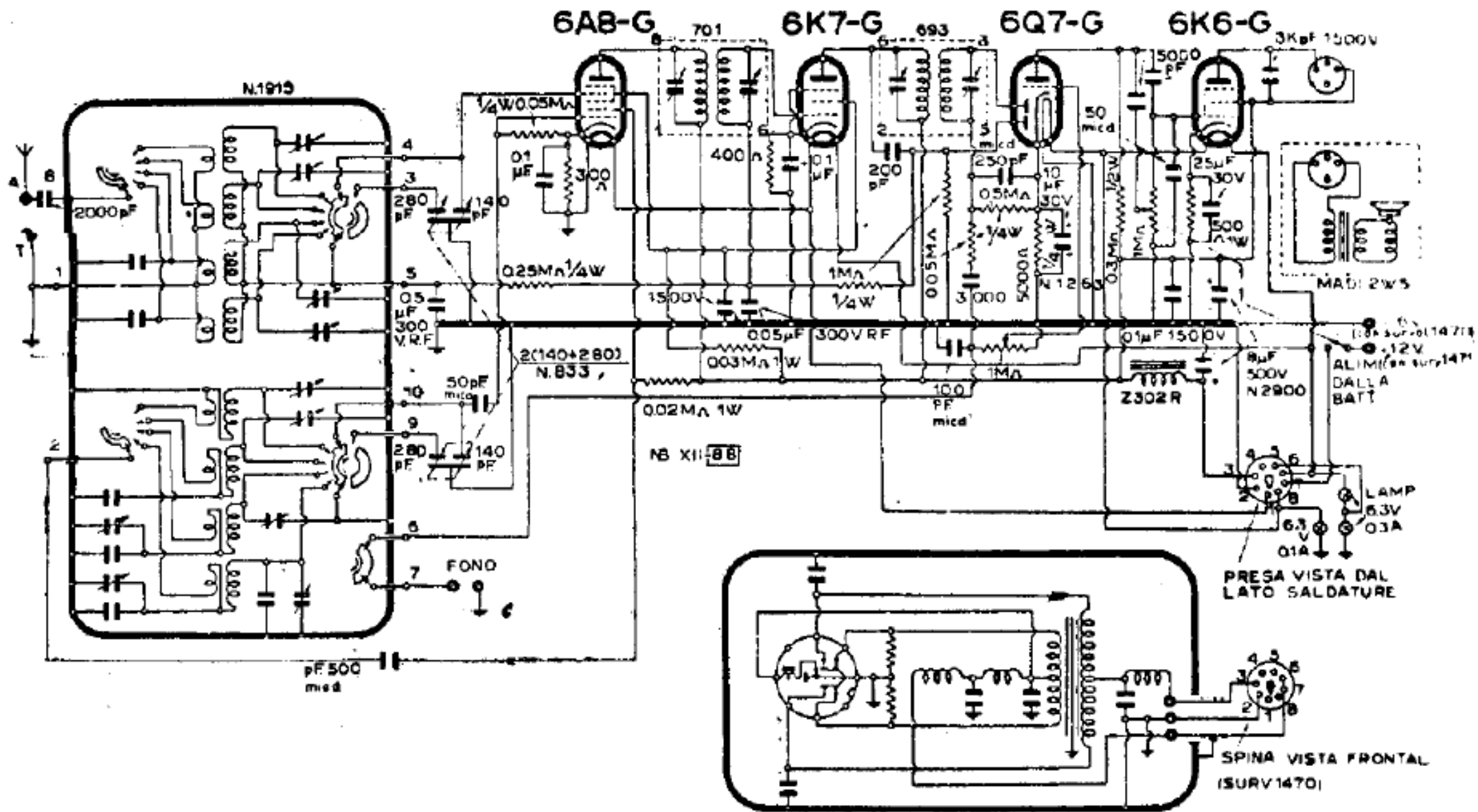
GELOSO (SOC.) - MOD. SUPER « G 49/A »
